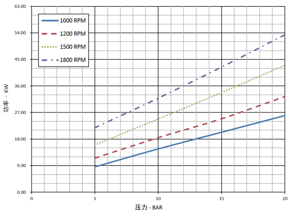
功率vs. 排出压力-水
