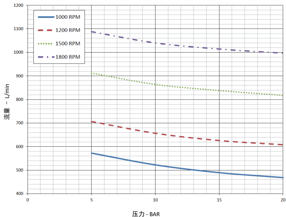
流量vs. 排出压力-水
